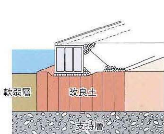
河川築堤、護岸等の基礎
